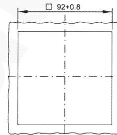
Otwór instalacyjny
